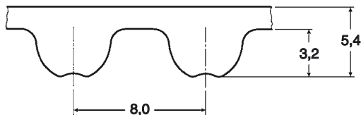
8M HP (nur Mittelwerte nominal dimensions – mm)
