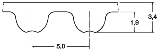
5M HP (nur Mittelwerte nominal dimensions – mm)
